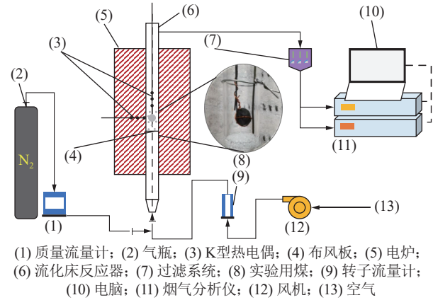
图 1 流化床煤燃烧实验流程
