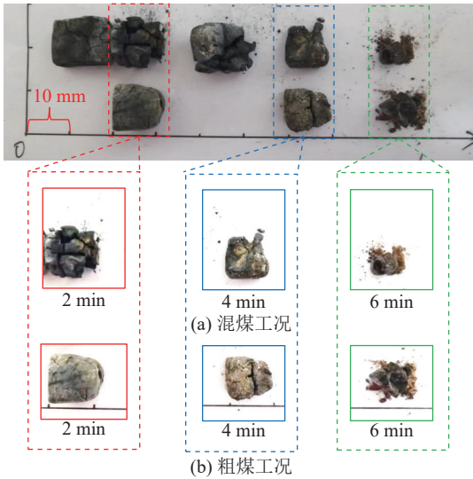
图4 不同燃烧时间内焦炭外貌
