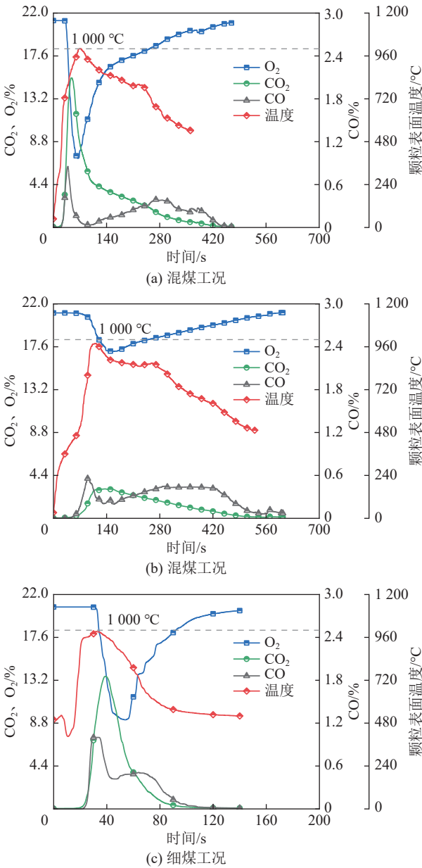
图 2 烟气组分及颗粒表面温度变化曲线
