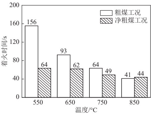
图 6 不同温度下各工况的着火时间
