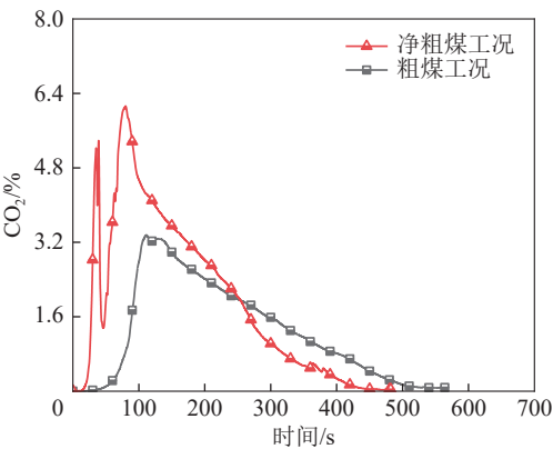
图 3 各工况的 CO 2 浓度曲线
