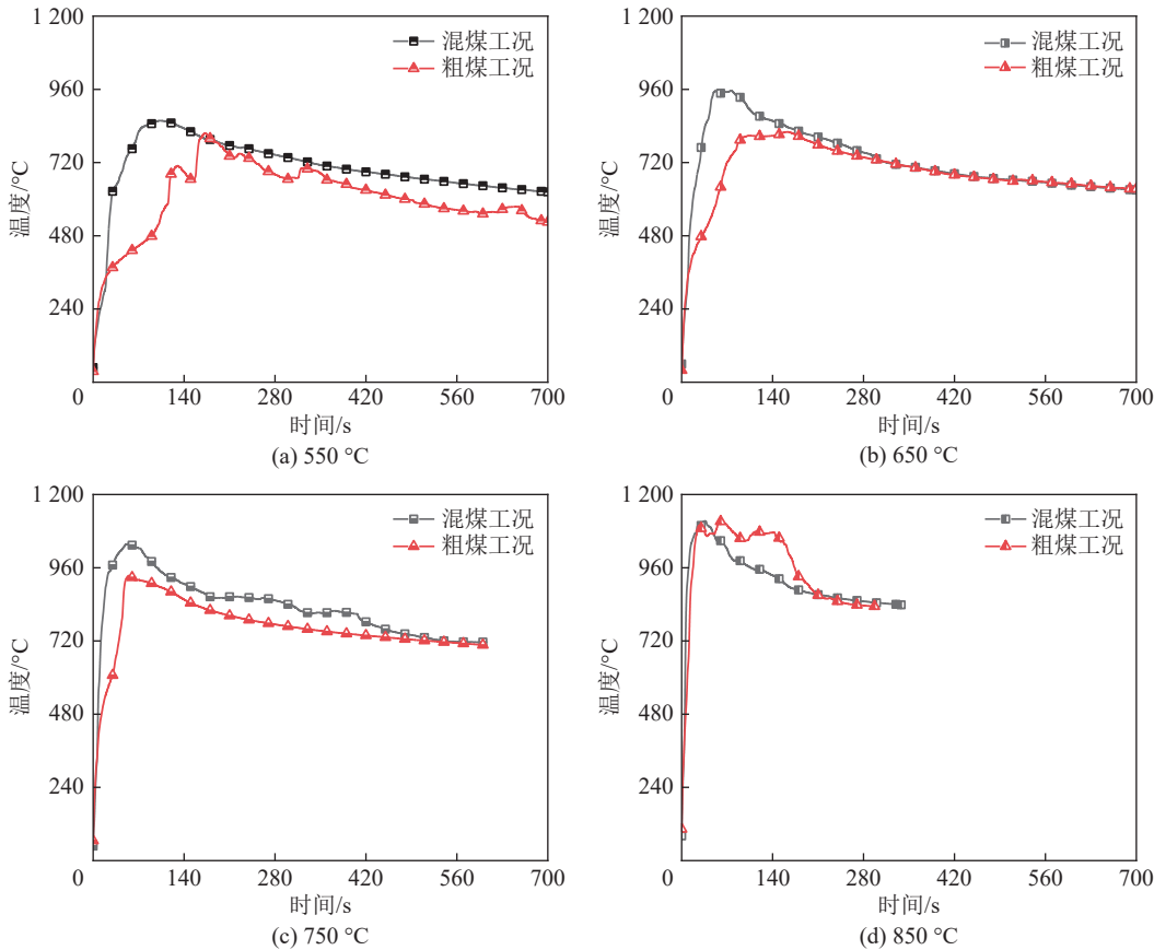
图 7 不同温度下各工况的颗粒温度
