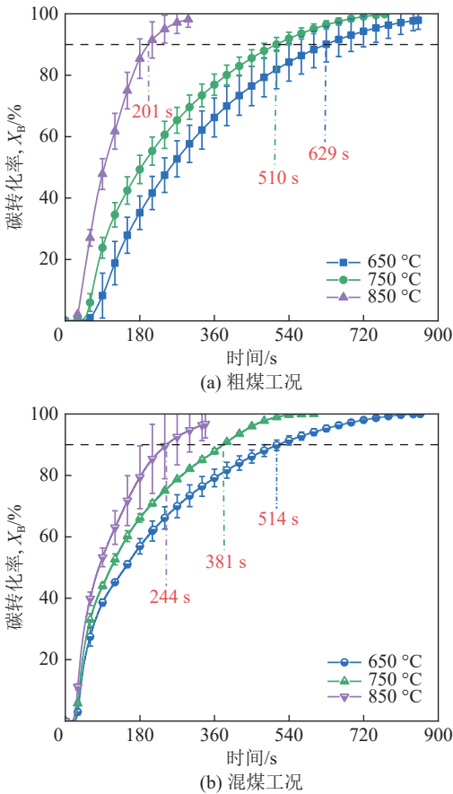
图5 不同温度下2个工况的转化率曲线
